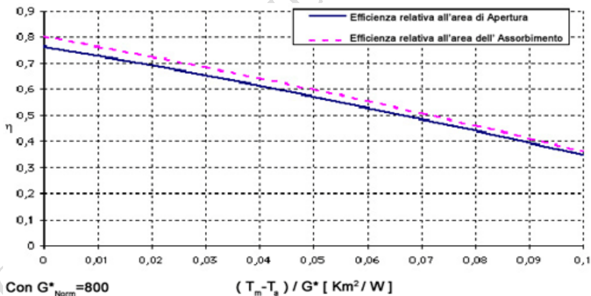
Grafico rendimento collettore solare
